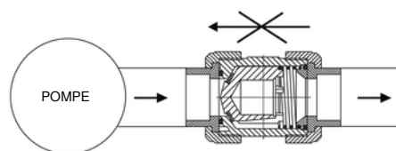
Fonction anti-retour
