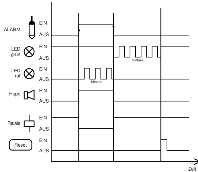
Fall 1: Alarm kommt und verschwindet wieder von alleine (zum Beispiel durch Wellenbewegung der Flüssigkeitsoberfläche), die blinkende grüne LED wird danach mit der RESET-Taste quittiert.
