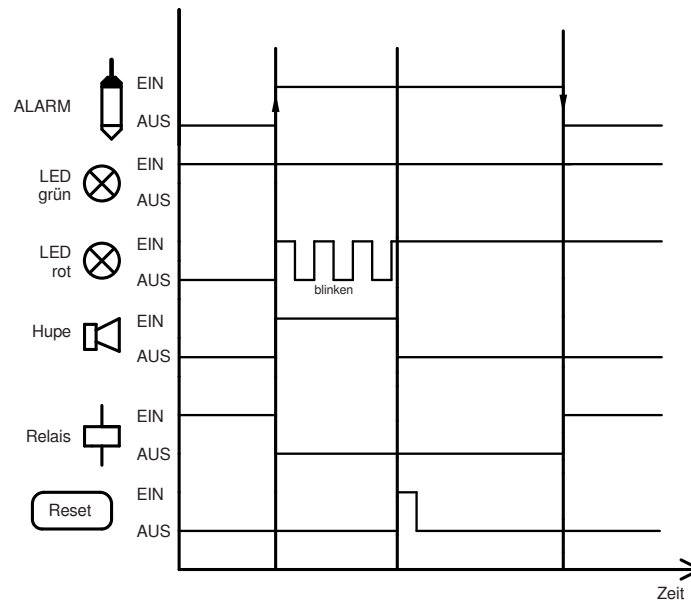
Fall 2: Alarm kommt und steht → Reset wird gedrückt, Alarm wird quittiert, nach Beseitigung der Alarmursache geht die rote LED wieder aus.
