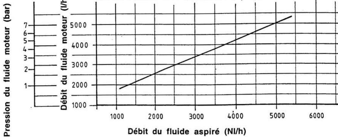
AVEC PERCAGE DE LA BUSE : \varnothing 7 mm
