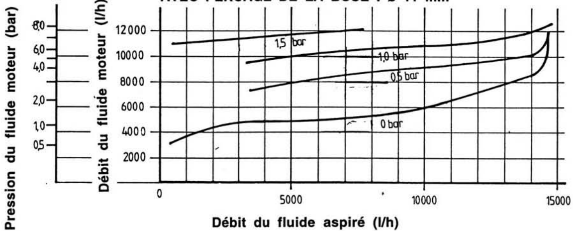
AVEC PERCAGE DE LA BUSE : \varnothing 11 mm
