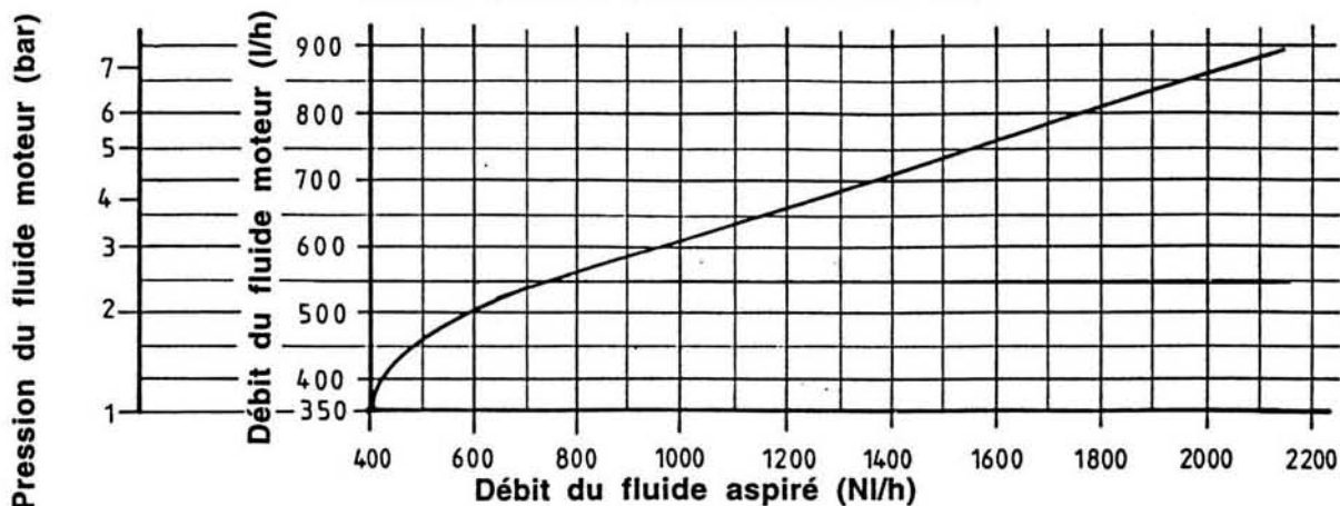
AVEC PERCAGE DE LA BUSE : \varnothing 3 mm
