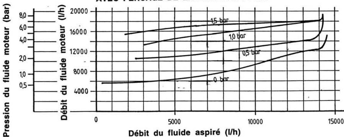
AVEC PERCAGE DE LA BUSE : \varnothing 14 mm
