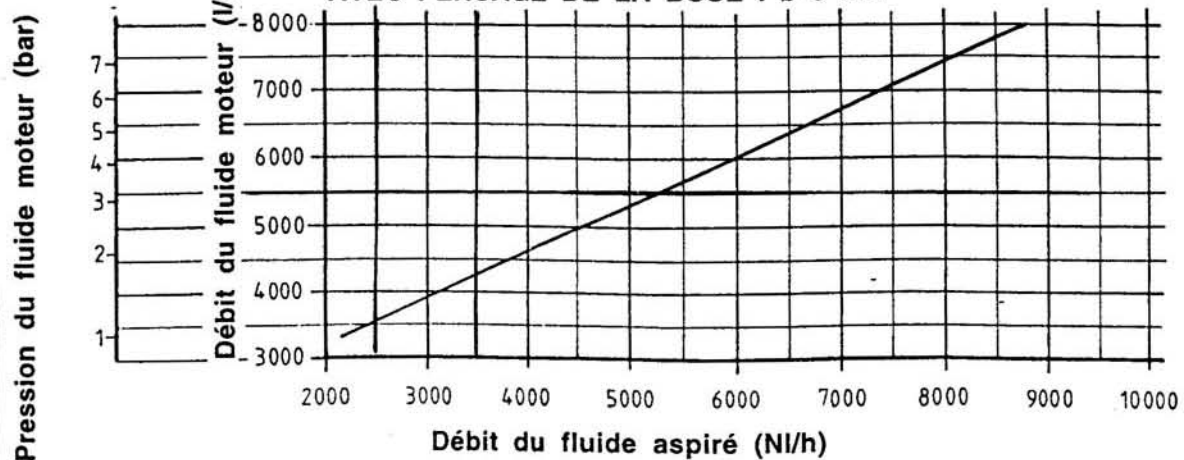
AVEC PERCAGE DE LA BUSE : \varnothing 9 mm
