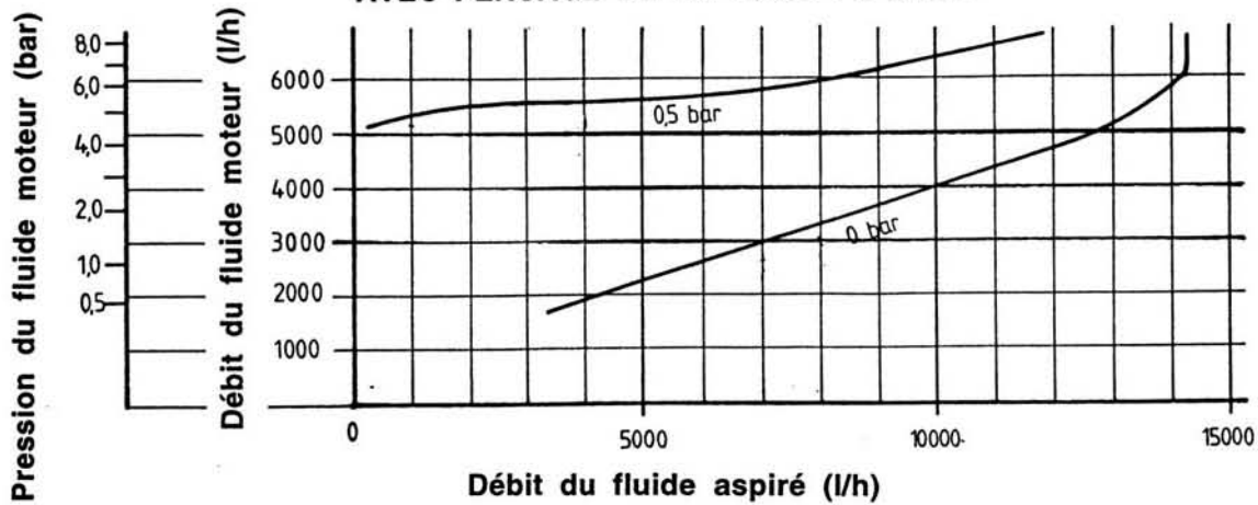
AVEC PERCAGE DE LA BUSE : \varnothing 8 mm
