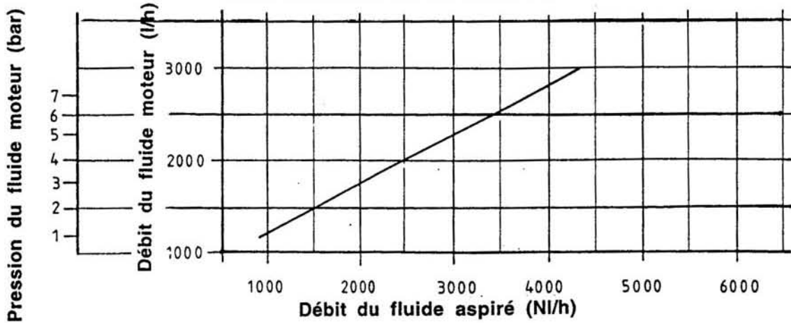
AVEC PERCAGE DE LA BUSE : \varnothing 5 mm
