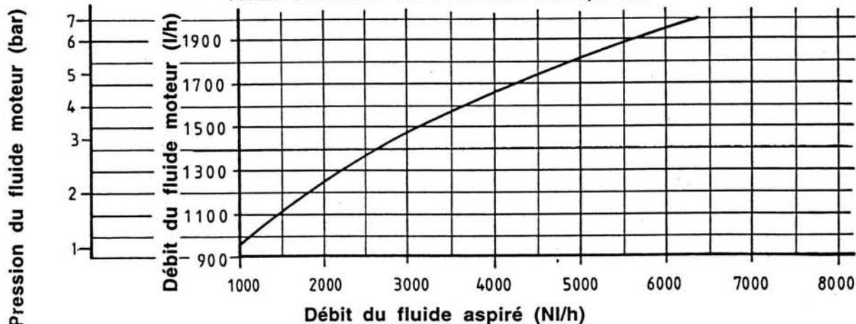
AVEC PERCAGE DE LA BUSE : \varnothing 4,5 mm
