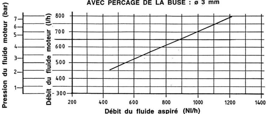
AVEC PERCAGE DE LA BUSE : \varnothing 3 mm
