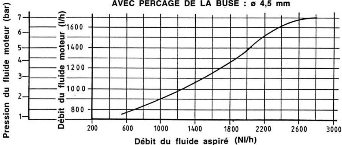
AVEC PERCAGE DE LA BUSE : \varnothing 4,5 mm
