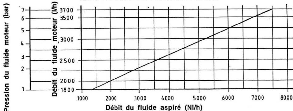
AVEC PERCAGE DE LA BUSE : \varnothing 6 mm
