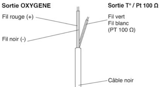
Raccordement Sonde BAMOX 7200 sur BAMOPHOX
