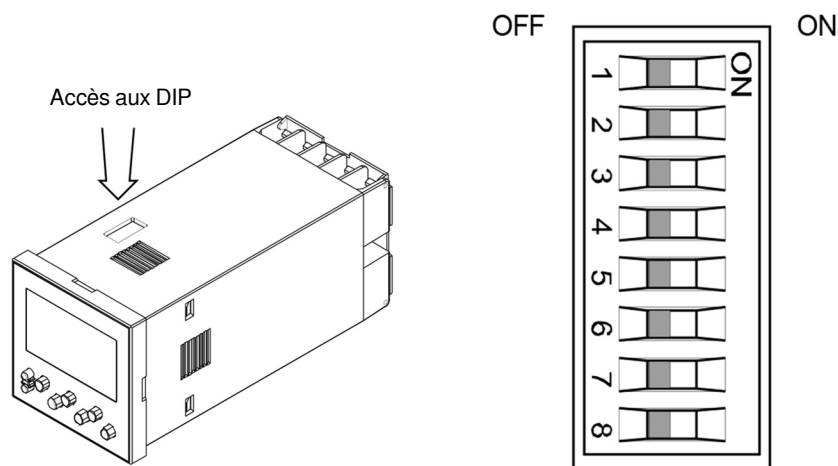
Fig. 7.1 Commutateurs DIP
