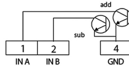
Collecteur ouvert
