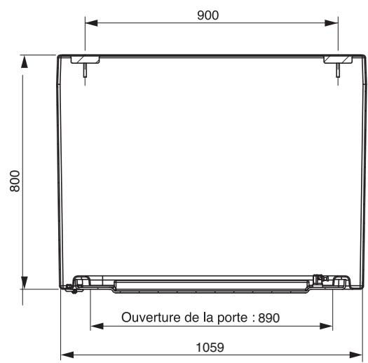
Coupe B-B
